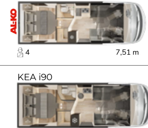
4 7,47 m
